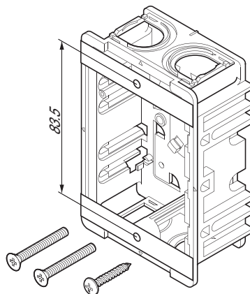
⑤ スライドボックス (付属:十字穴付皿小ねじM4×40 2本 十字穴付トランペットドリリング タッピンねじ3.8×32 1本)
