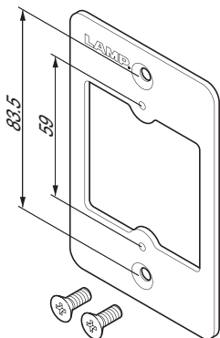
④ スペース (付属:十字穴付皿 小ねじM4×12 2本)
